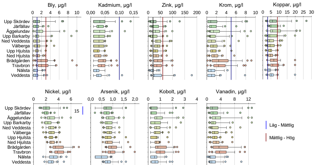
Figur 33. Metaller, ofiltrerade, µg/l. Månatliga provtagning 2019 och 2022. 10, 25, 50 (median), 75 och 90 percentiler. Röd linje = medelvärde. Gränser är angivna för Låg till Måttlig och Måttlig till Hög halt enligt NV Rapport 4913.
