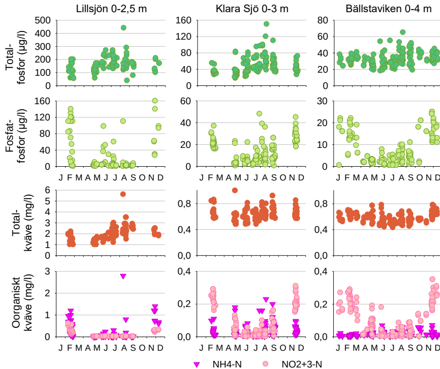
Figur 49. Totalfosfor och fosfatfosfor, totalkväve och oorganiskt kväve (ammonium- och nitrit+nitratkväve) i Lillsjön, Klara Sjö och Bällstaviken, variation under året, samtliga värden 2013-2022. NB olika skalor.
