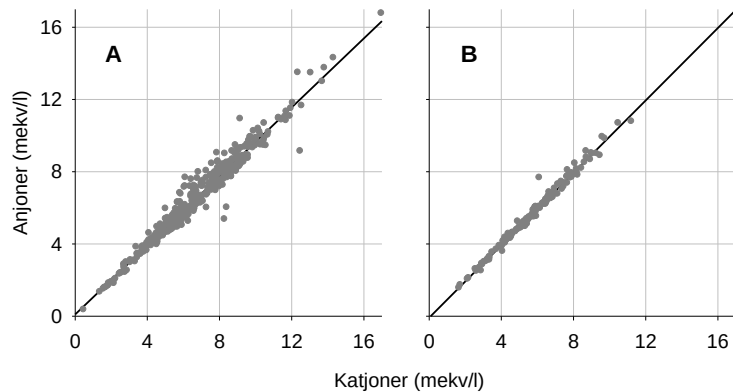
Figur 13. Samband mellan an- och katjoner, (A) Bällstaåns huvudfåra 2018-2022 och (B) SLU:s provtagningar vid Travbron 2012-2022.
