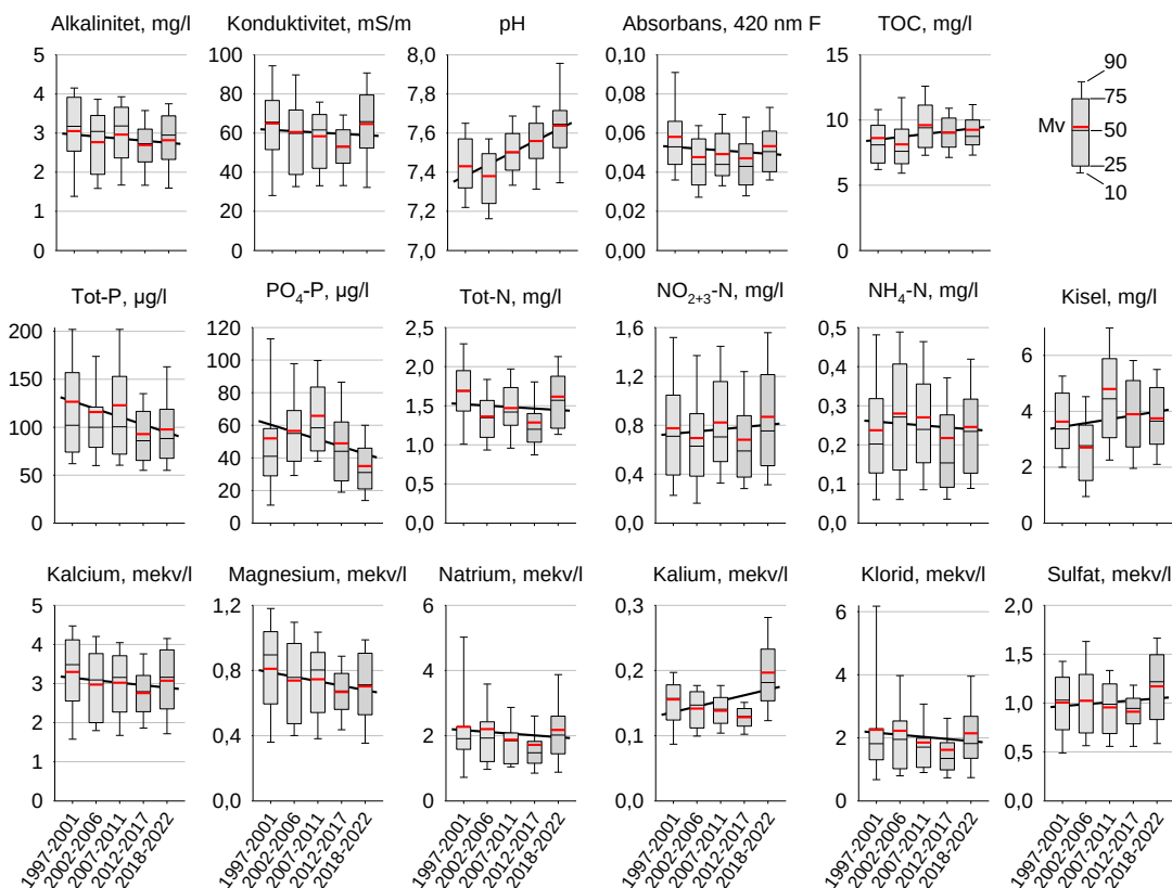
Figur 37. SLU, provtagningar i Bällstaåns mynning, 1997-2011 nedströms och 2012-2022 uppströms Solvalla. Grupperade mätvärden, 10, 25, 50 (median) 75 och 90-percentiler samt medelvärden (röd linje).
