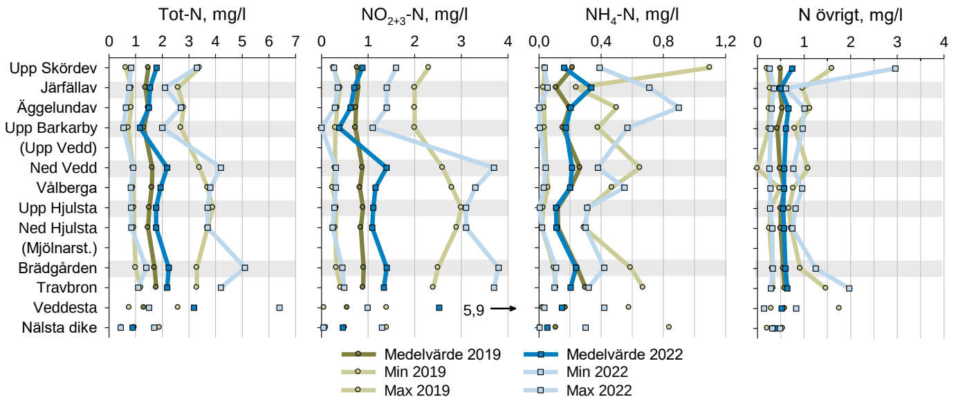
Figur 19. Totalkväve, nitrit+nitratkväve och ammoniumkväve samt "övrigt" kväve i Bällstaån 2019 och 2022; medelvärden, min och maxvärden.
