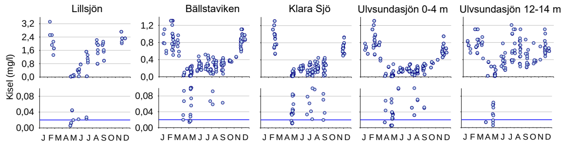
Figur 55. Kisel, mg/l, årsvariation i Lillsjön 1919-2022, Bällstaviken och Klara Sjö samt Ulvsundasjön 2013-2022, samtliga värden utom Ulvsundasjön medelvärden 0-4 m och 12-14 m. Undre diagrammen med förstord skala, blå linje anger sannolikt begränsande halt, 0,02 mg/l. NB olika skalor.
