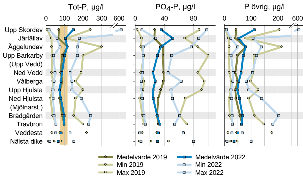
Figur 16. Totalfosfor, fosfatfosfor och övrig fosfor i Bällstaån 2019 och 2022; medelvärden, min och maxvärden. Koncentrationsområde för Otillfredsställande halt av totalfosfor (76-115 \mu\text{g/l} ) är angivet med brun färg.
