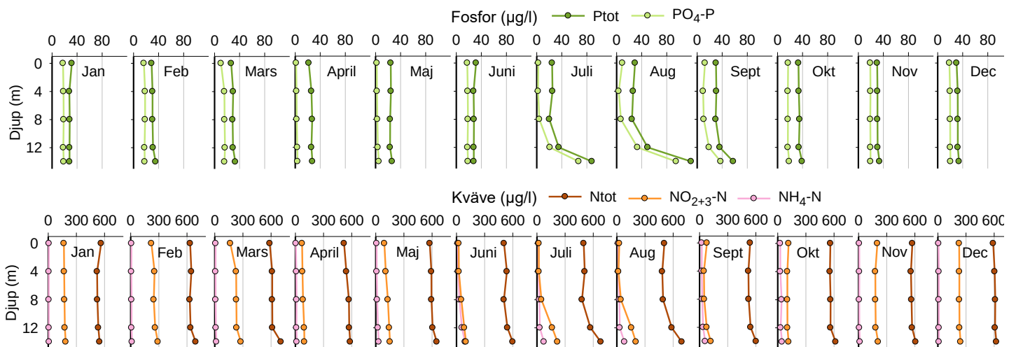
Figur 50. Fördelningen av fosfor (fosfat- och totalfosfor) och kväve (ammonium-, nitrit+nitratkväve och totalkväve) på 0-14 m djup i Ulvsundasjön, medelvärden respektive månad 2000-2020.
