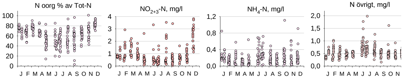
Figur 18. Kväve, årsvariation 2019 och 2022. Oorganiskt kväve som procent av totalkväve samt halter av nitrit+nitratkväve, ammoniumkväve och "övrigt" kväve.
